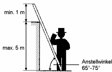
Anstellwinkel und min. Länge für Anlegeleitern
